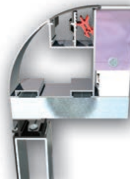
детайл на монтажа на разделителя
